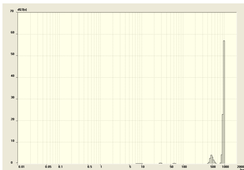
Рис. 1. Размеры частиц (ось абсцисс) и их доля (в %) (ось ординат) во взвеси из района «пляж МорГУ» без включения ультразвука
